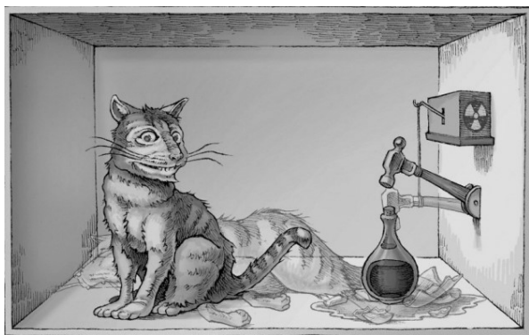
图 3 著名的薛定谔猫悖论示意图
