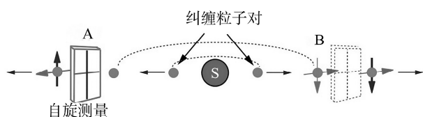
图 2 EPR 纠缠粒子对的测量示意图
